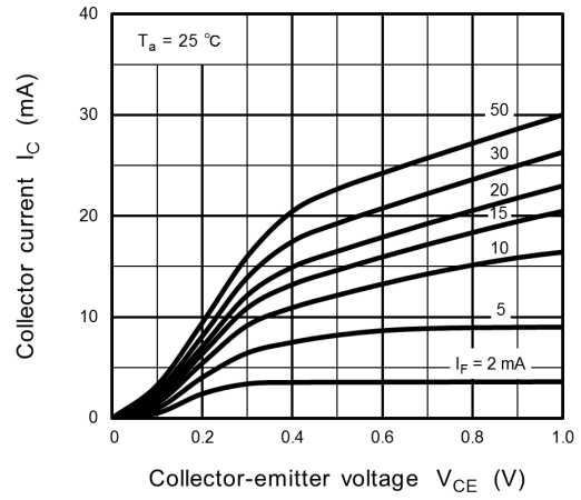
Fig. 11.8 I_C - V_{CE0}
