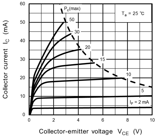
Fig. 11.7 I_C - V_{CE0}
