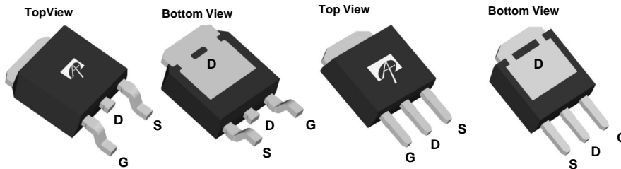
TO252 DPAK: AOD516
