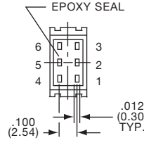
P.C. HOLE LAYOUT DOUBLE POLE
