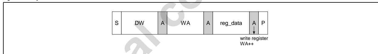
Figure 25. Byte Write
